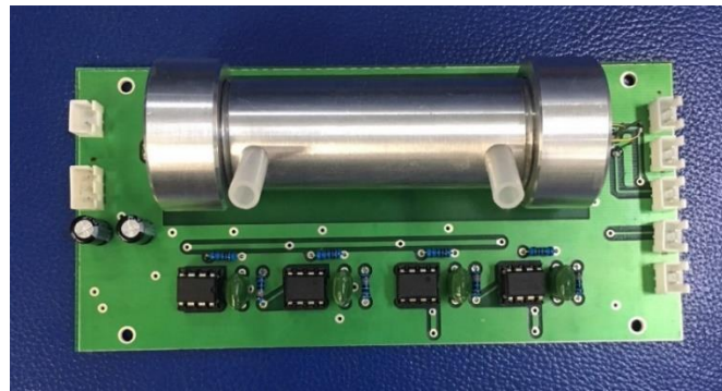
Hình 1. Ảnh chụp thiết bị đã chế tạo về cảm biến theo cấu hình NDIR
