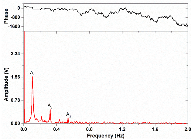
Hình 4. Kết quả minh họa biến đổi Fourier nhanh (FFT) của một bộ số liệu điện áp U_{\text{Thermopile}}
