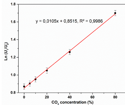
Hình 5. Đường chuẩn hóa tín hiệu của hai kênh thu \ln(U_1/U_2) phụ thuộc vào nồng độ khí CO_2
