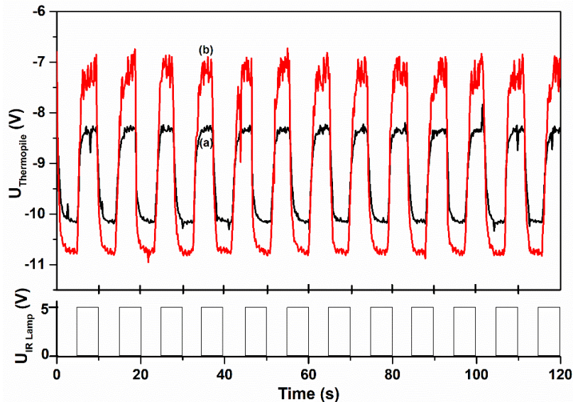
Hình 3. Các đường điện áp U_{Thermopile} của kênh so sánh (a) và kênh nhạy khí (b) theo thời gian tương ứng với chu kỳ điện áp cấp cho đèn hồng ngoại U_{IR-Lamp}
