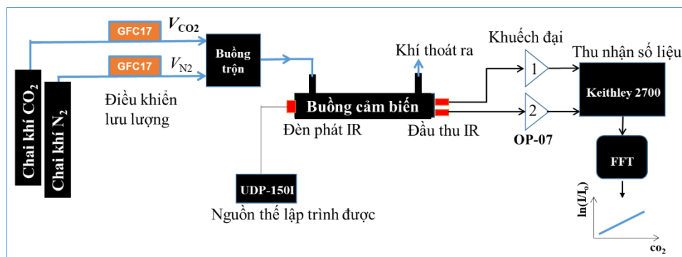
Hình 2. Sơ đồ thiết kế cho phân tích nồng độ khí chuẩn CO 2 bằng cấu hình cảm biến hấp thụ hồng ngoại NDIR sử dụng biến đổi FFT
